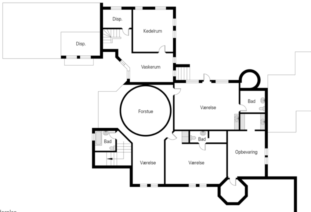
Kælderplan Plantegning er ikke målfast.
